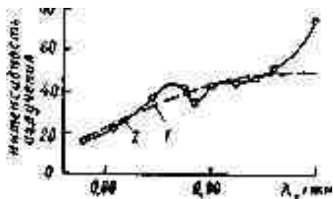
Рис. 12.11. Кривые спектрального распределения энергии, излучаемые: 1 — АЧТ при 2850 К; 2 — пламенем вспышки фотобомбы М-120, снаряженной фотосмесью
