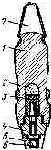
Рис. 15.5. Бронебойно-зажигательно-трассирующий снаряд:
