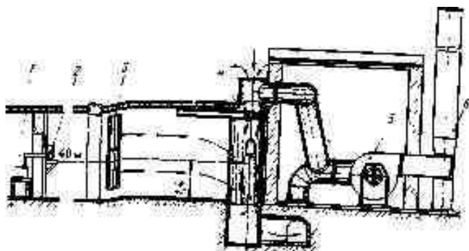
рис. 11.21. Схема фотометрической камеры:
