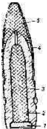
Рис. 15.4. Бронебой-но-зажигательный снаряд:
