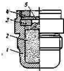
Рис. 13.5. Трассер:
