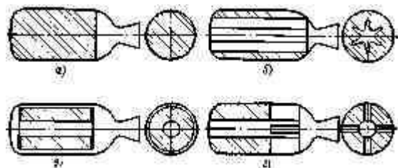
Рис. 18.7. Типичные формы зарядов твердого топлива:
