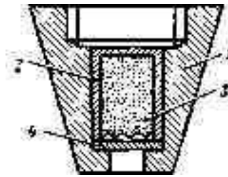
Рис. 13.7. Трассер к взрывателю МД-5:
