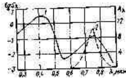
Рис. 12.4. Кривые спектральной чувствительности (Л) и фотоакти-нического потока ( A\lambda ) под красным светофильтром КС-14 (2) инфра-хроматической аэрофотоплёнки
