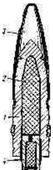
Рис. 15.6. Бронебойно-зажигательно-трассирующий снаряд'
