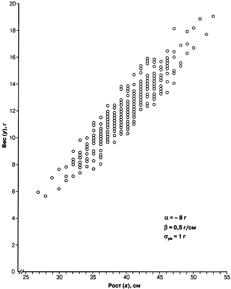
Рис. 8.1. Рост и вес марсиан. Как известно, число обитателей Марса составляет 200; каждый из них был измерен и взвешен, результат нанесен на график в виде кружка. Распределение марсиан по росту и по весу нормально. Более того, средний вес марсиан определенного роста связан с ростом линейной зависимостью; разброс значений веса для всех ростов одинаков. Чтобы к совокупности можно было применить регрессионный анализ, она должна обладать всеми этими свойствами.
