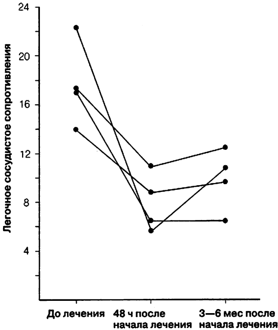
Рис. 9.6. Изменение легочного сосудистого сопротивления у 4 больных с легочной гипертонией при лечении гидралазином.
