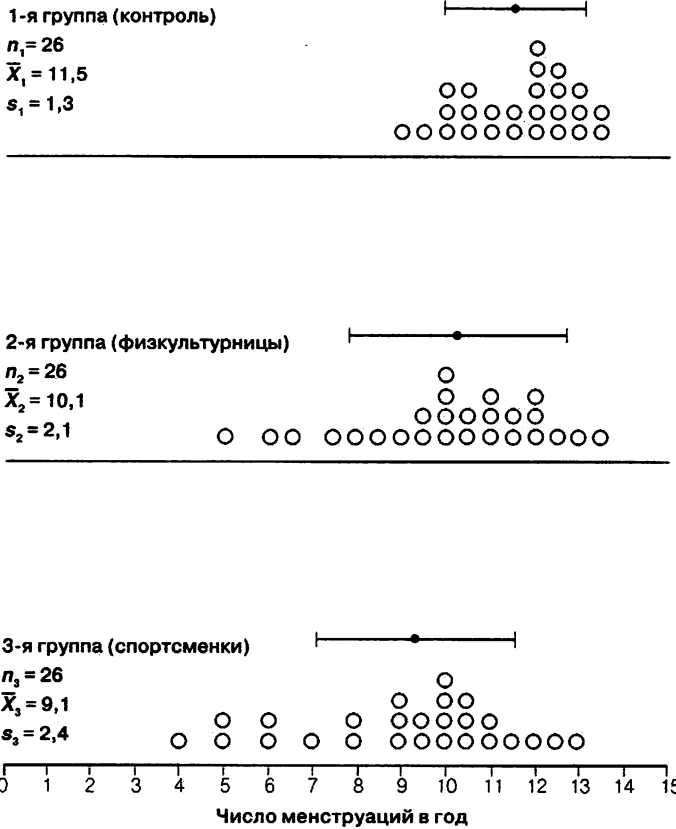
Рис. 3.9. Число менструации в год у женщин которые не занимались ни физкультурой, ни спортом (1-я группа), физкультурниц (2-я группа) и спортсменок (3-я группа). Среднее число менструаций различно. Можно ли отнести эти различия за счет случайности.
