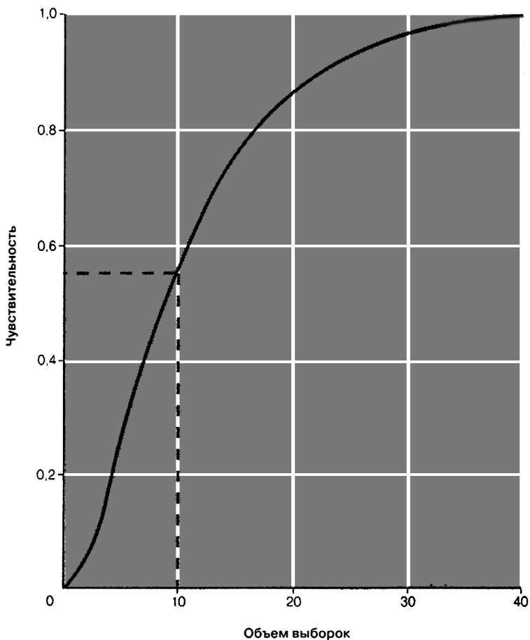
Рис. 6.8. Чувствительность критерия Стьюдента как функция от объема выборок при величине различий 200 мл, уровне значимости \alpha = 0,05 и стандартном отклонении \sigma = 200 мл. При объеме выборок 10 человек чувствительность составляет 0,55.
