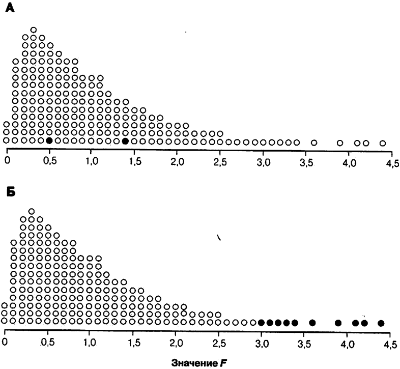
Рис. 3.6. А. Четыре случайные выборки по 7 человек в каждой извлекли из той же совокупности (население городка) 200 раз. Каждый раз рассчитывали значение F и наносили его на график. Результаты для выборок с рис. 3.2 и 3.5 помечены черным. Б. Десять наибольших значений помечены черным. Область черных кружков начинается со значения F , равного 3,0.
