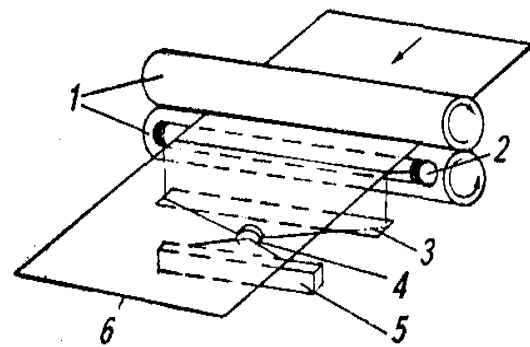
Рис. 5.3.5. Схема роликового сканера: 1— ролики подачи бумаги; 2—лампа; 3— зеркало; 4— объектив; 5 — светочувствительный элемент; 6—оригинал
