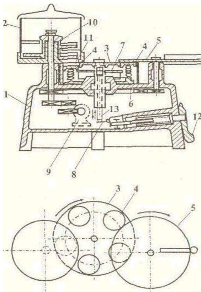
Рис. 9. Котлетный автомат
