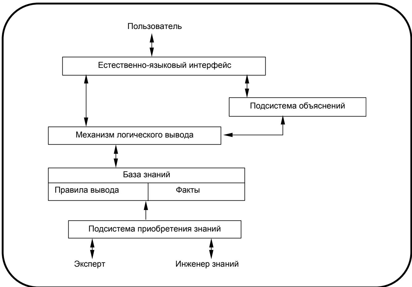
Рис. 3.13. Структура экспертной системы
