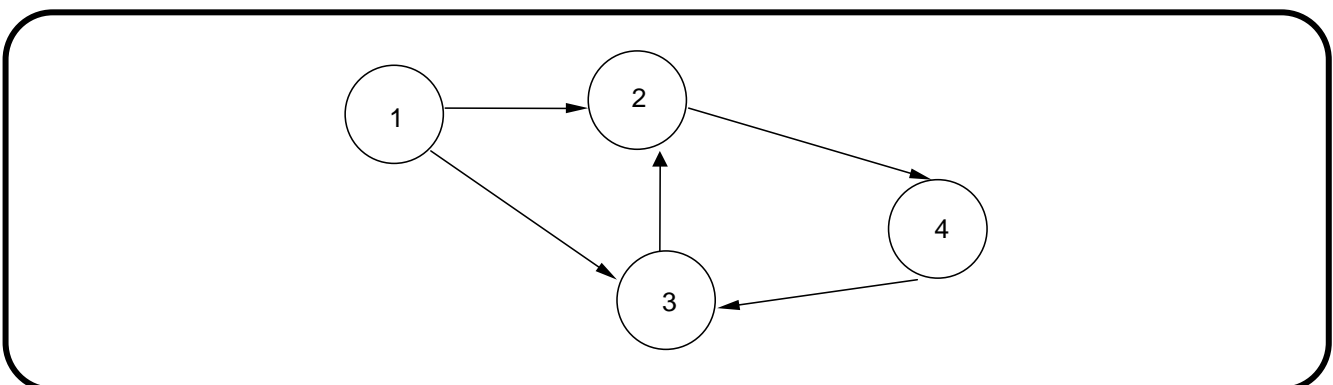
Рис. 3.7. Пример орграфа с контуром
