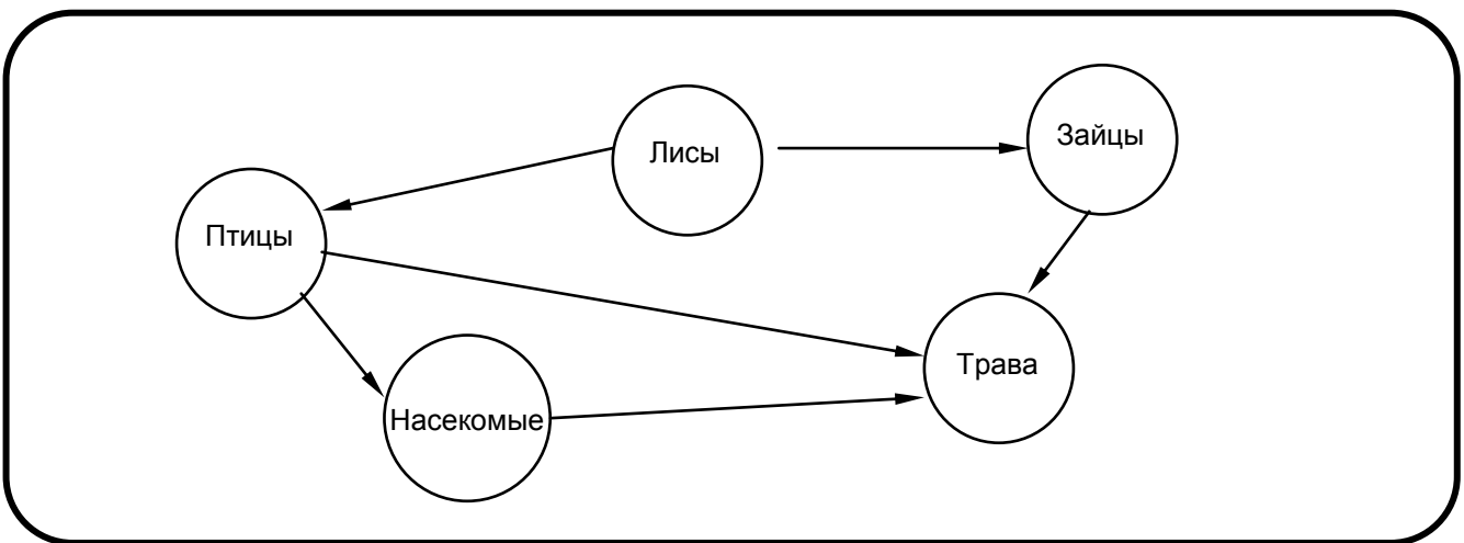
Рис. 3.10. Сеть питания для пяти живых организмов
