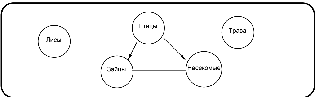
Рис. 3.11. Граф конкуренции для сети питания, представленной на рис. 3.10
