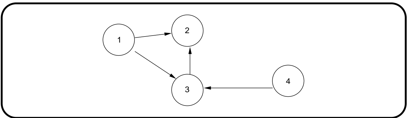
Рис. 3.6. Пример ориентированного графа
