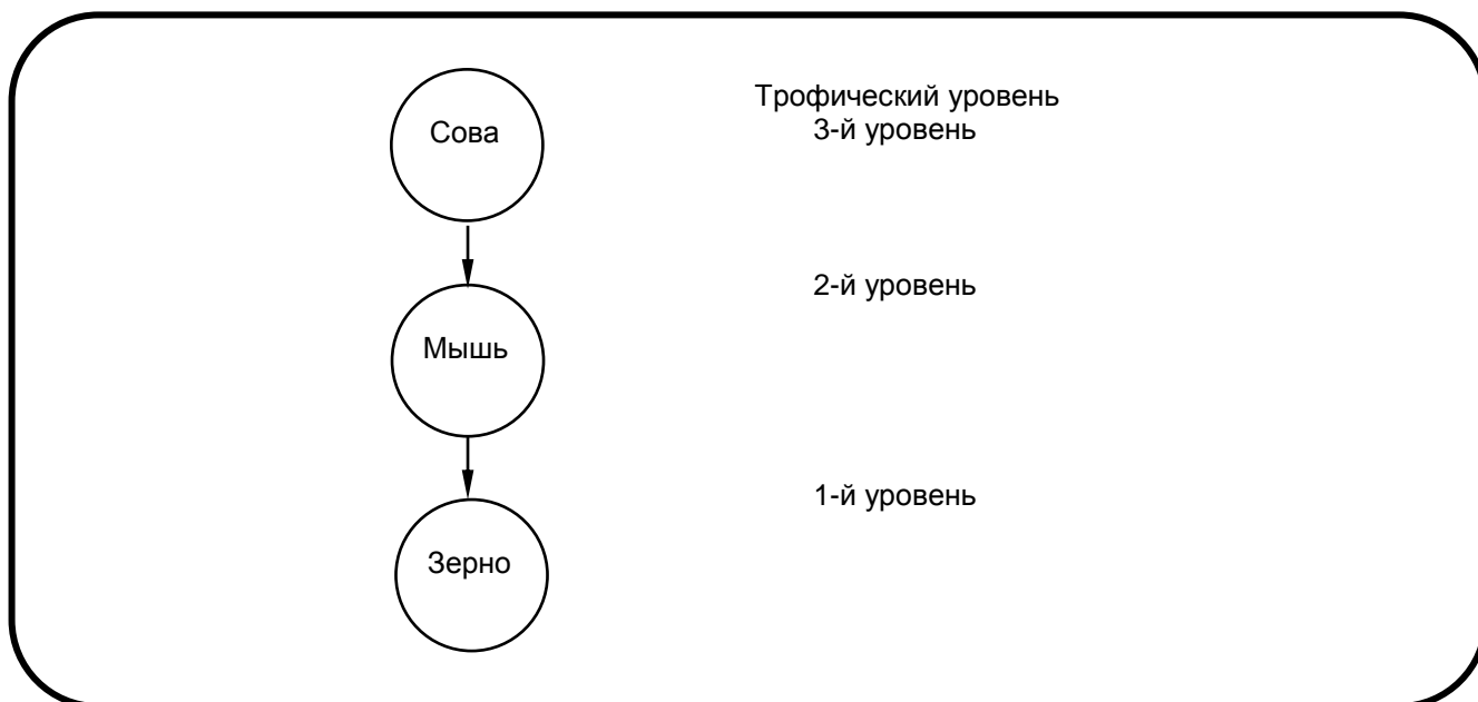
Рис. 3.12. Пищевая цепь, представляющая однозначное определение трофического уровня
