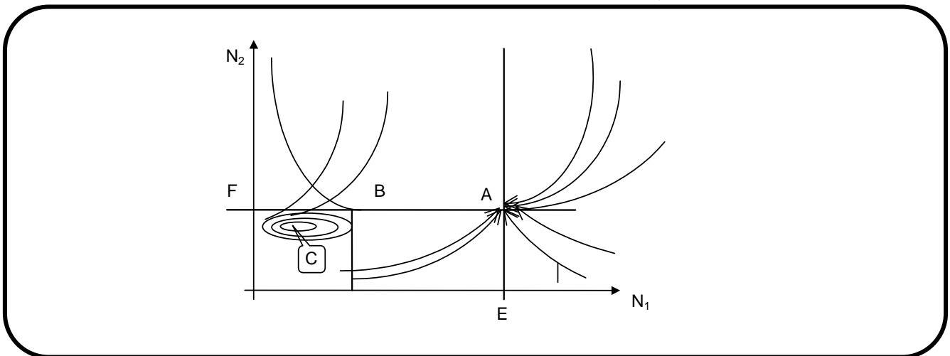
Рис. 3.5. Общая картина всех фазовых точек
