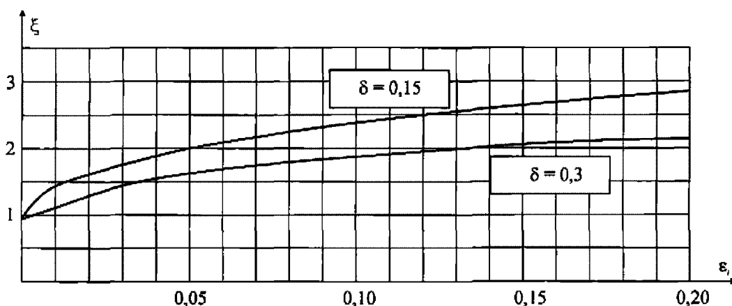
Рисунок 11.1 - Коэффициенты динамичности
