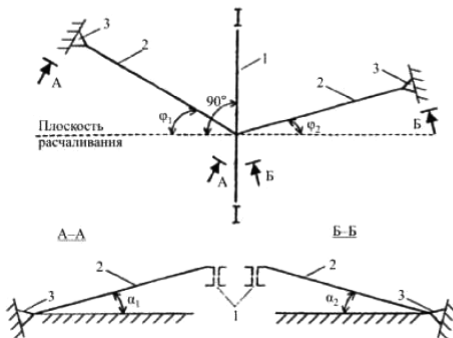
Рисунок К.2 - Схема раскрепления ферм расчалками
